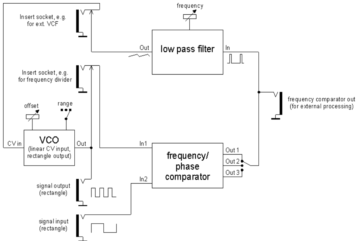
Abb. 1: Blockschaltbild des A-196
